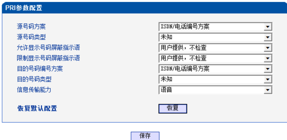
图 2-5-2 PRI 参数
