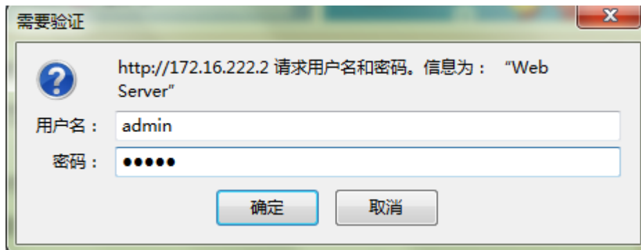
图 2-1-1 登录界面
